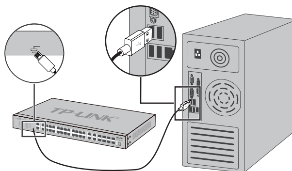
图3-4 Micro USB Console端口连接示意图
